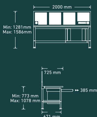
Stół warsztatowy WB 630
